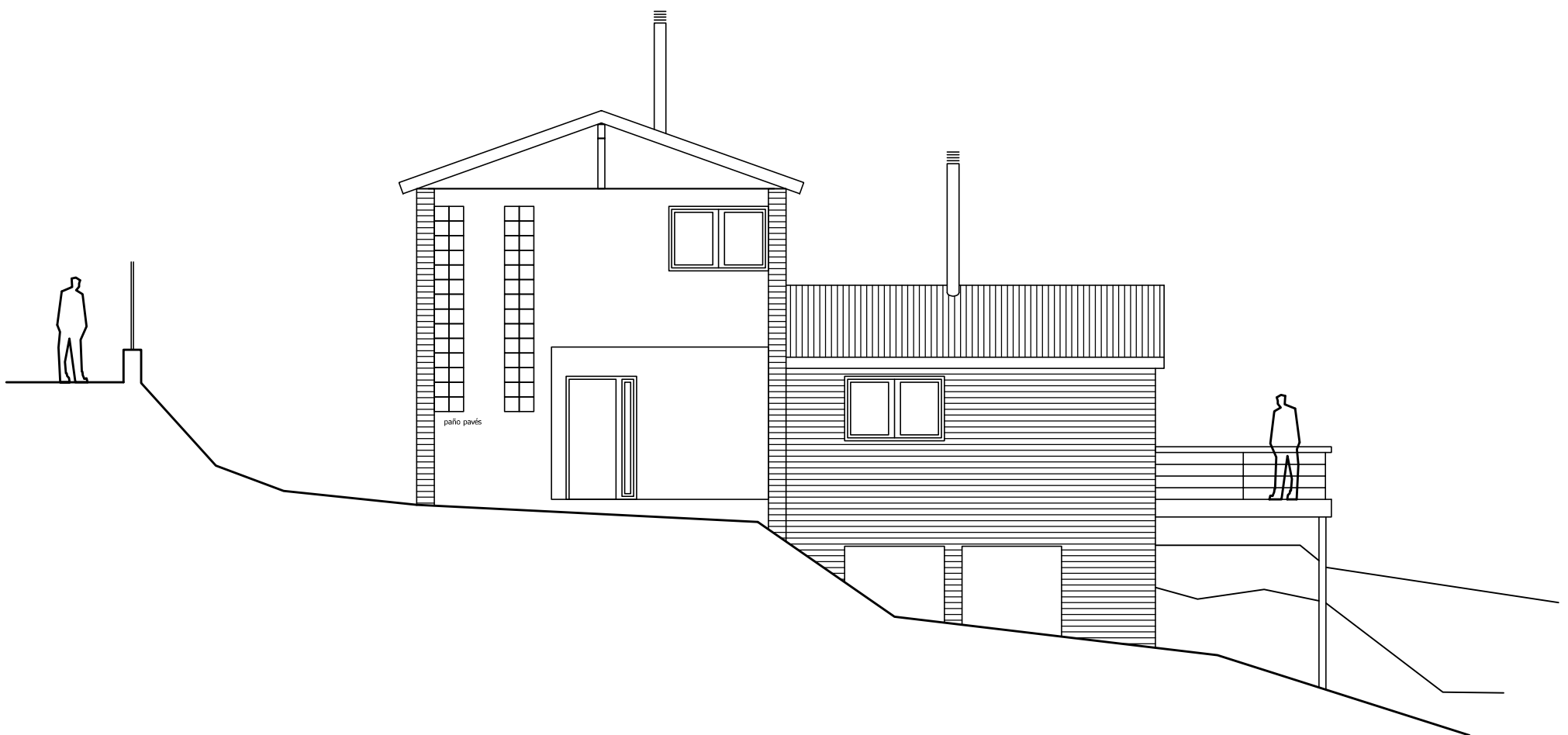
alzado sur
